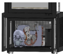
Figura 17: Unidade Condensadora
