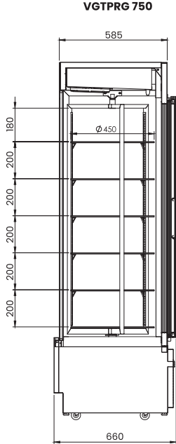
VITRINE GLASS TOWER PREMIUM PRATELEIRA GIRATÓRIA 750
