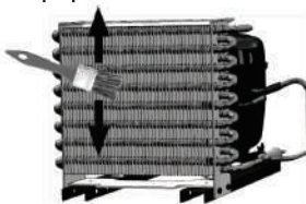
Figura 15: Limpando o condensador
