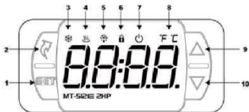
Figura 5: Termostato MT512E
