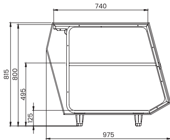
PESAGEM AÇOUGUE ATLANTIS
