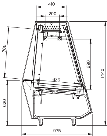
EXPOSITOR AÇOUGUE ATLANTIS GANCHEIRA
