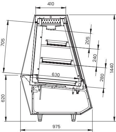
EXPOSITOR AÇOUGUE ATLANTIS PRATELEIRAS
